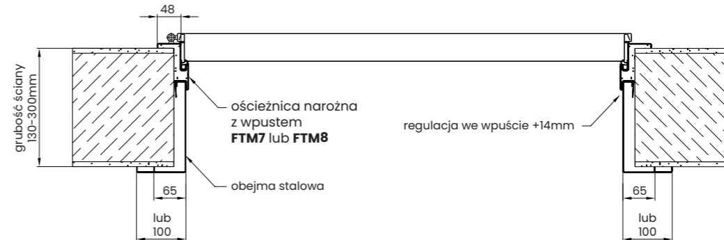
PRZEKRÓJ POZIOMY
