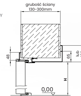
PRZEKRÓJ PIONOWY
