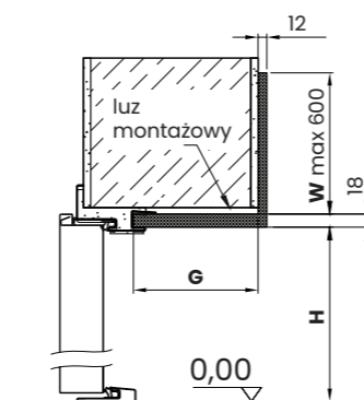
PRZEKRÓJ PIONOWY
