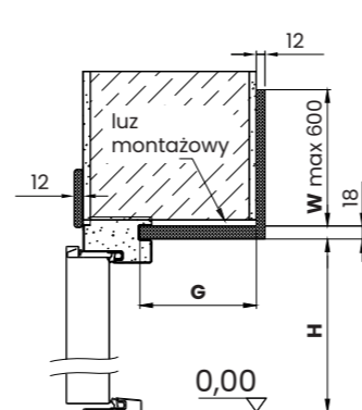
PRZEKRÓJ PIONOWY
