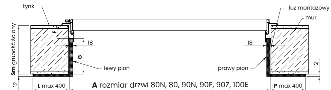
PRZEKRÓJ POZIOMY
