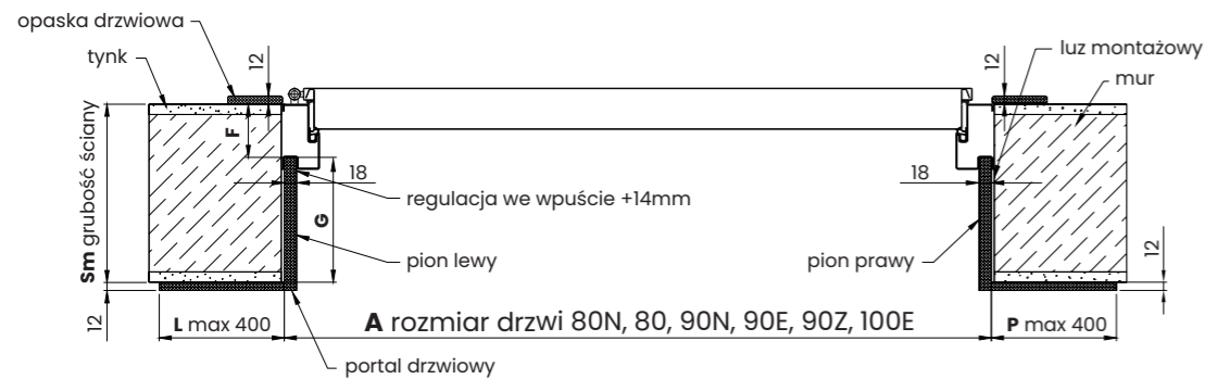
PRZEKRÓJ POZIOMY
